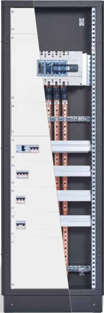
XL³ S 630 - her sırada 24 modül
